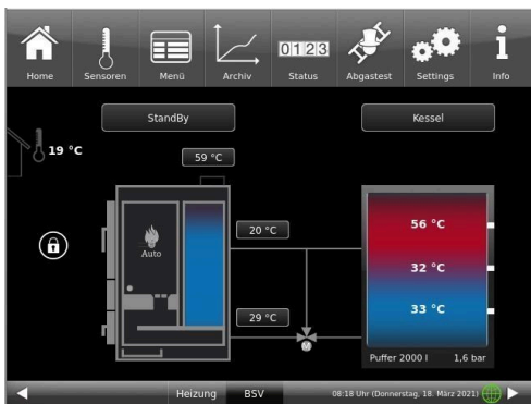
Abbildung 12: Schwarzes-Display-Design
