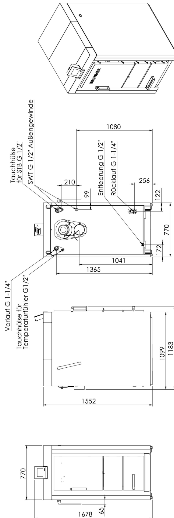
Abbildung 47: BSV 40 / BSV 50
