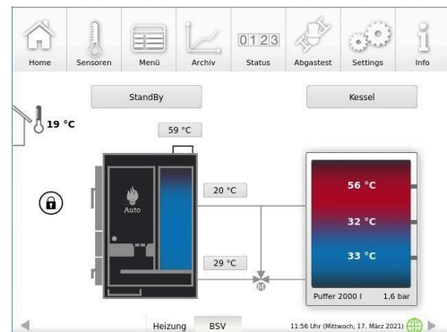
Abbildung 13: Weißes Display-Design
