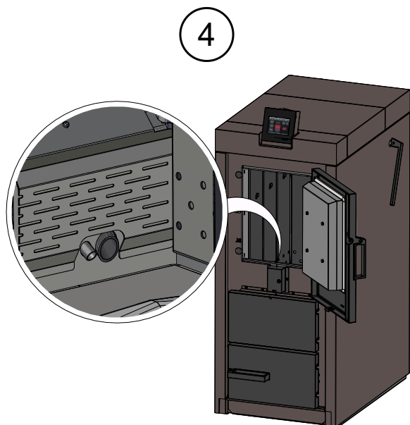
Abbildung 41: Zünderrohr
